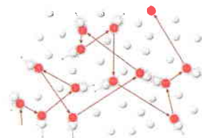
Mișcarea browniană Figura I.1
